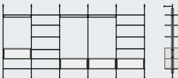
COMPOSIZIONE 6 COMBINATION 6 463 x 53 x h 240 cm 172" x 21" x h 94"
