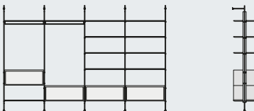
COMPOSIZIONE 4 COMBINATION 4 370 x 53 x h 240 cm 146" x 21" x h 94"
